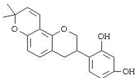
Glabridin
