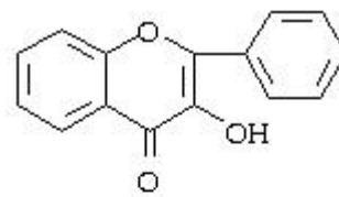
Flavonol
