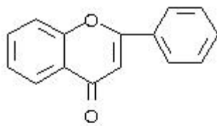
Flavon
